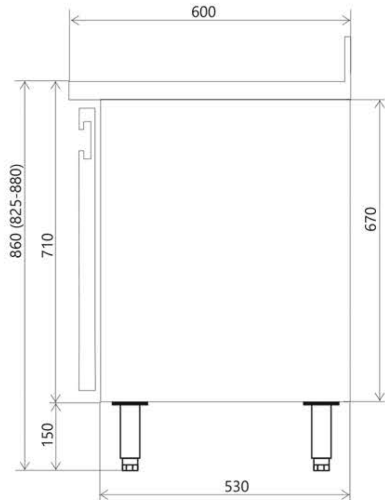
Side SK+SP
